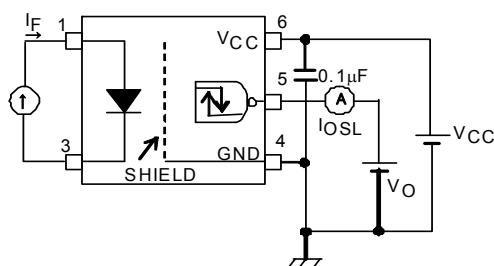
Test Circuit 5 : I_{OSL}
